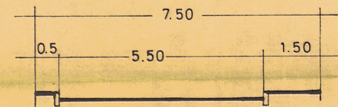
Strassenprofil M 1:100
